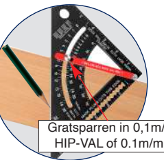
Markieren von Gratsparren Marking of HIP-VAL
